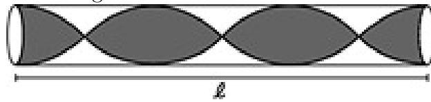
Figura 3.8: Tubo harmônico 3.
