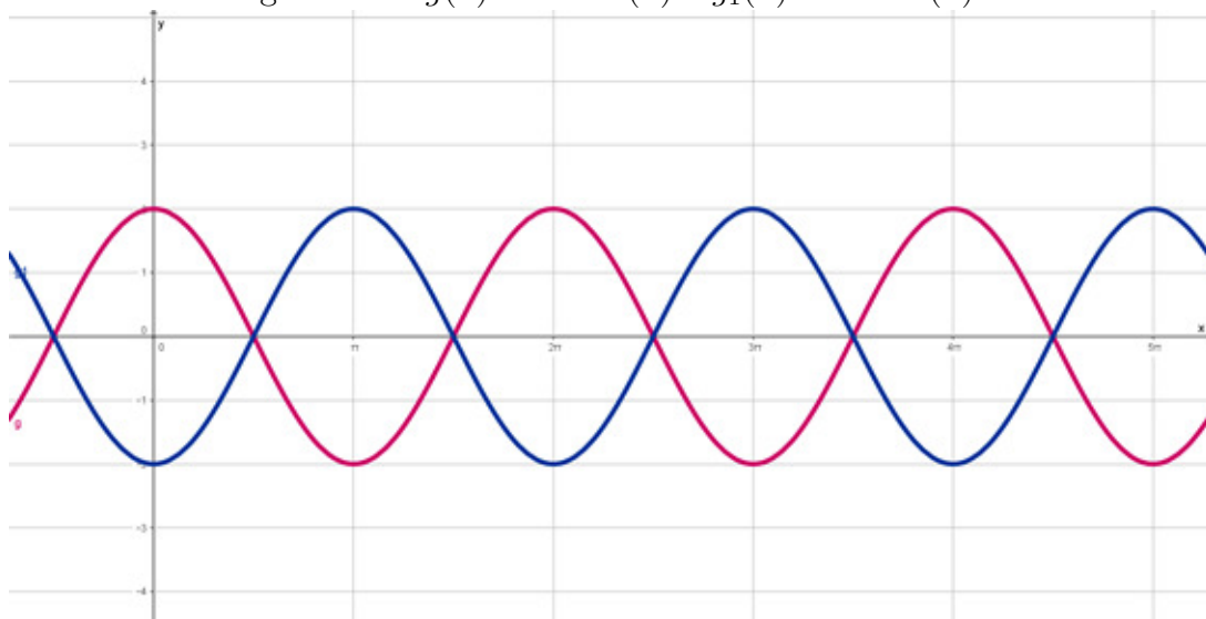
Figura 5.11: g(x) = 2 \cdot \cos(x) e g_1(x) = -2\cos(x) .
