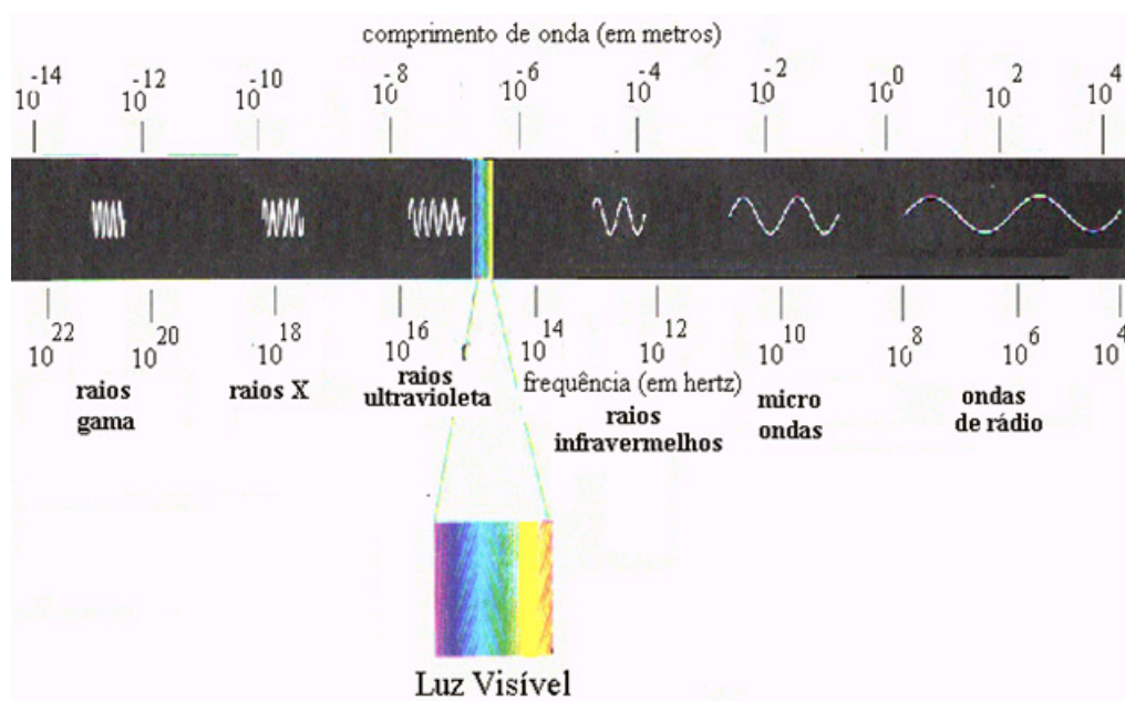
Figura 2.15: Espectro eletromagnético.
