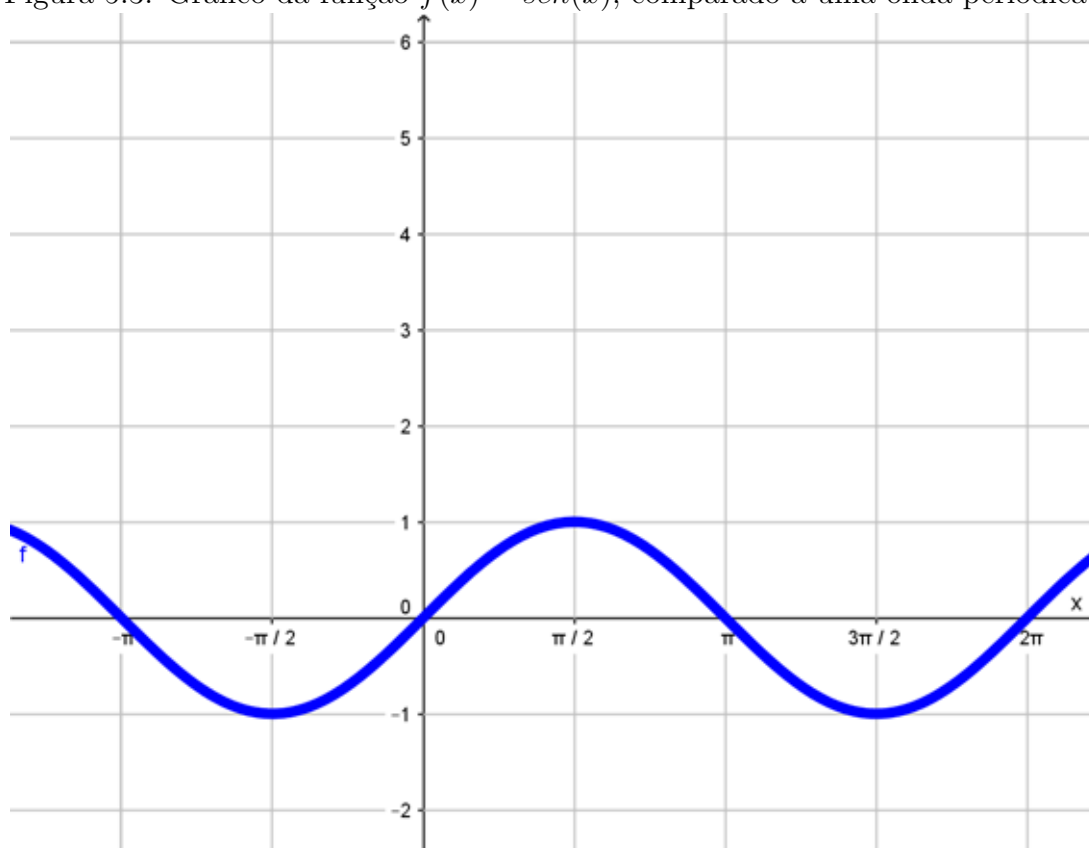
Figura 5.3: Gráfico da função f(x) = \text{sen}(x) , comparado à uma onda periódica.
