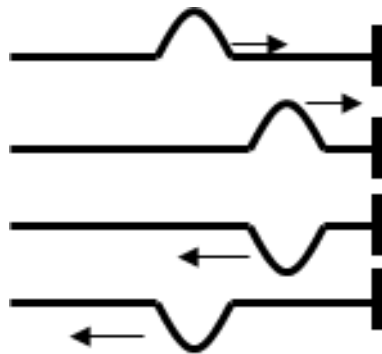
Figura 2.20: Ondas com extremidade fixa.
