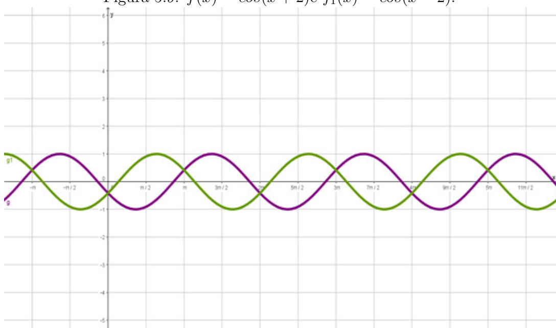
Figura 5.9: f(x) = \cos(x + 2) e f_1(x) = \cos(x - 2) .
