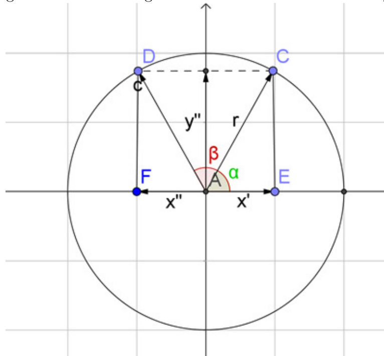
Figura 2.9: Círculo trigonométrico exibindo os arcos \alpha e \beta .
