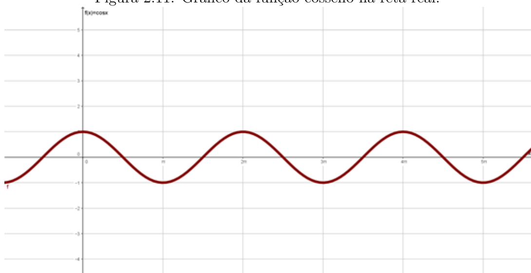
Figura 2.11: Gráfico da função cosseno na reta real.
