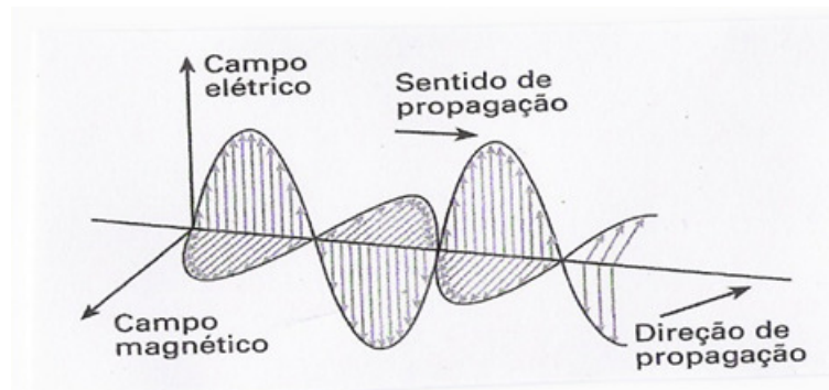
Figura 2.14: Ondas eletromagnéticas.
