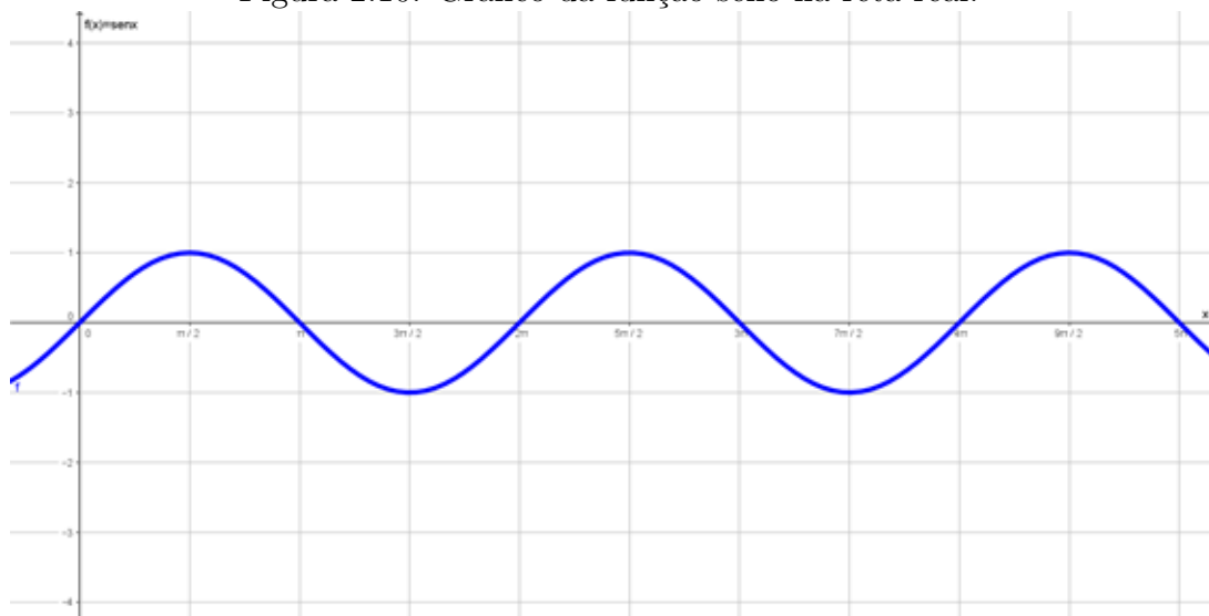
Figura 2.10: Gráfico da função seno na reta real.
