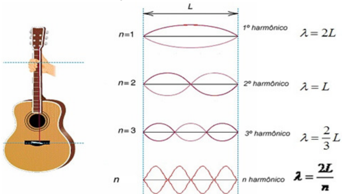
Figura 2.25: Ondas senoidais.
