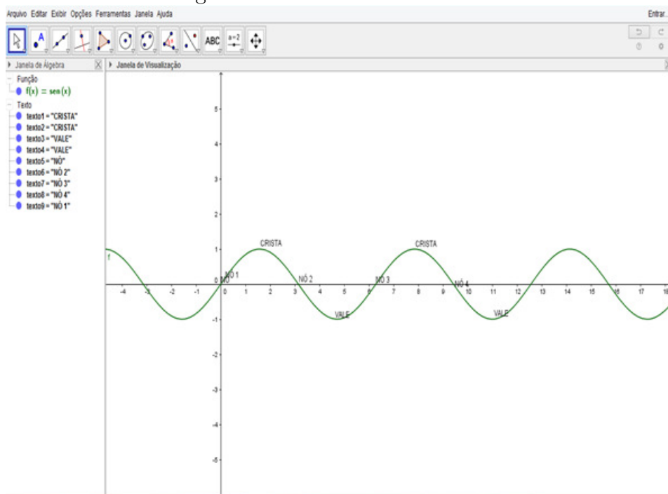
Figura 2.19: Ondas no GeoGebra.
