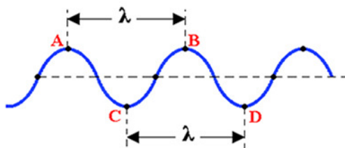
Figura 2.18: Ondas periódicas.
