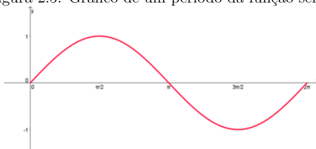
Figura 2.5: Gráfico de um período da função seno.
