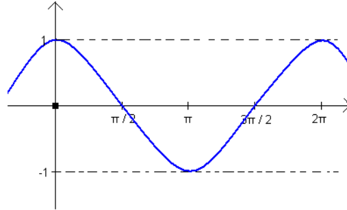
Figura 2.7: Gráfico da função cosseno.
