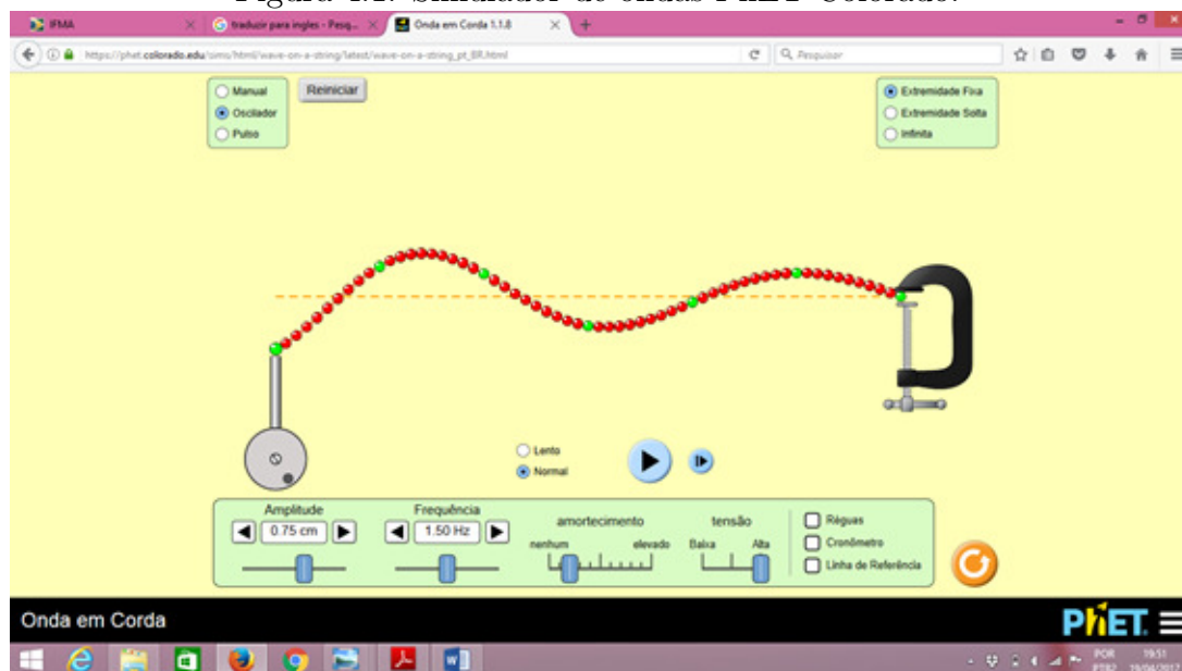
Figura 4.1: Simulador de ondas PhET Colorado.
