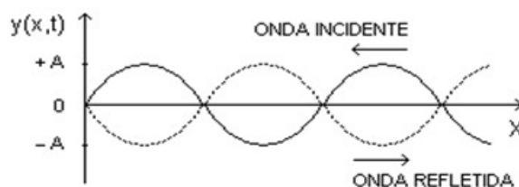
Figura 2.23: Onda estacionária.
