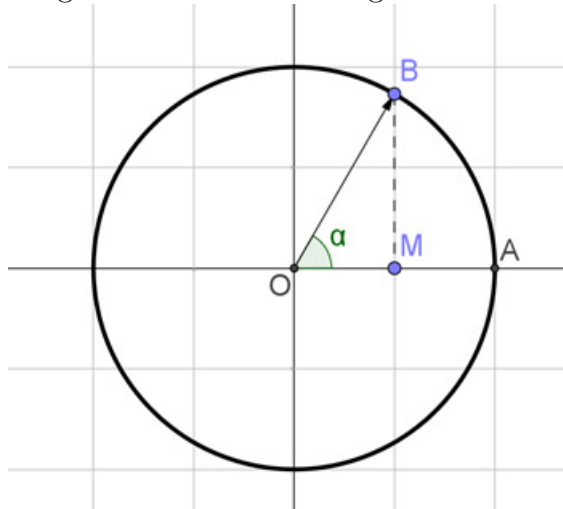
Figura 2.2: O Círculo trigonométrico.
