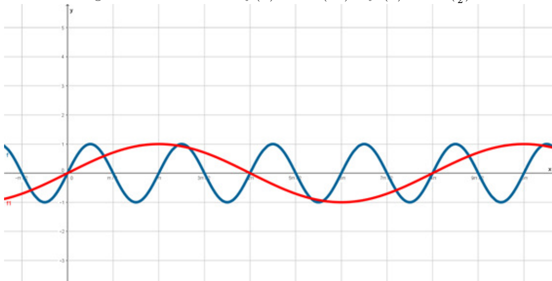
Figura 5.6: Gráficos de f(x) = \text{sen}(2x) e f_1(x) = \text{sen}(\frac{x}{2}) .
