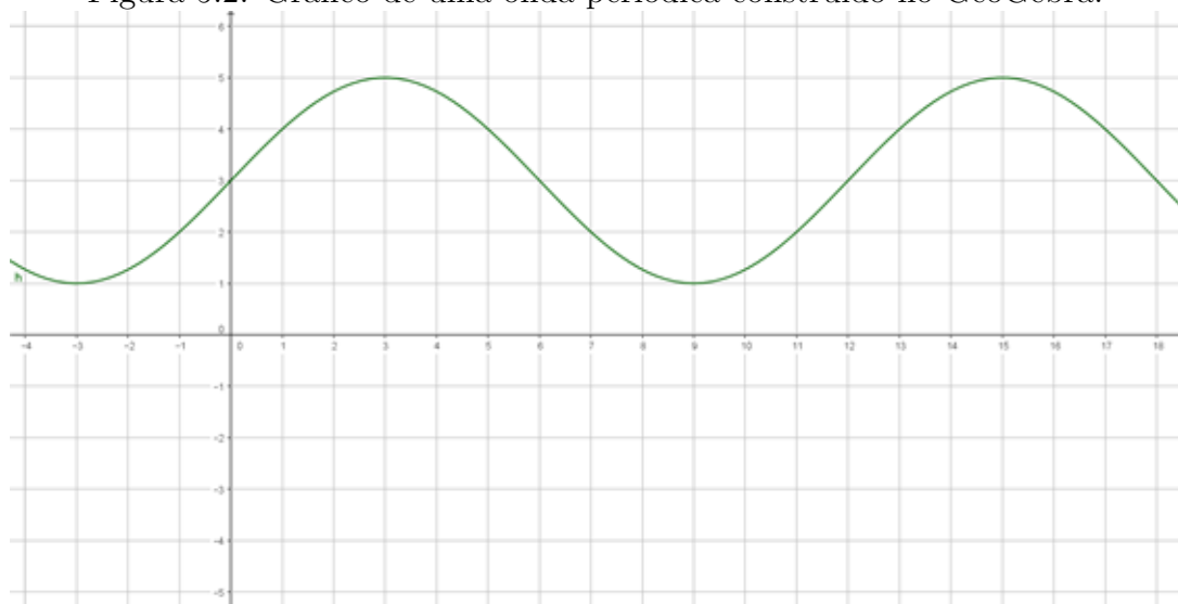
Figura 5.2: Gráfico de uma onda periódica construído no GeoGebra.
