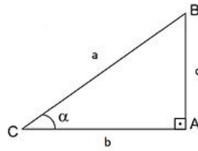
Figura 2.1: Triângulo Retângulo.
