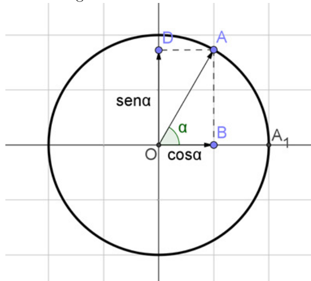
Figura 2.6: Ciclo trigonométrico exibindo o cosseno do ângulo x .
