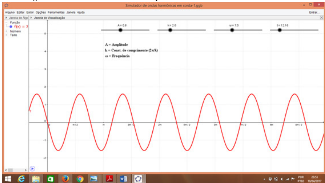
Figura 5.4: Simulador de ondas periódicas construído no GeoGebra.
