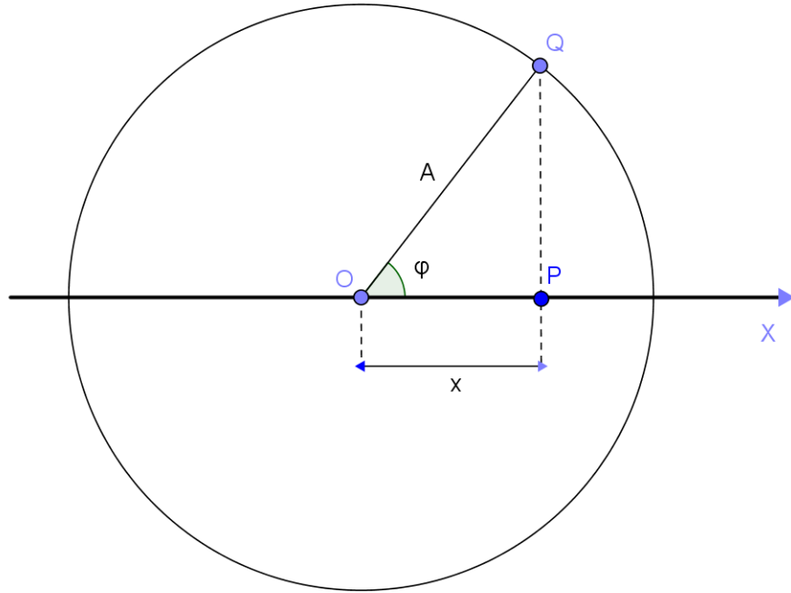
Figura 2.13: Projeção do M.C.U. no eixo horizontal.
