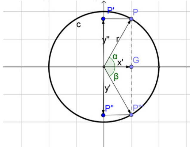
Figura 2.8: Ângulos simétricos.
