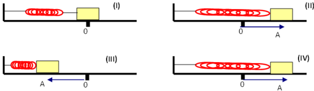
Figura 2.12: Oscilador Harmônico Massa-mola.
