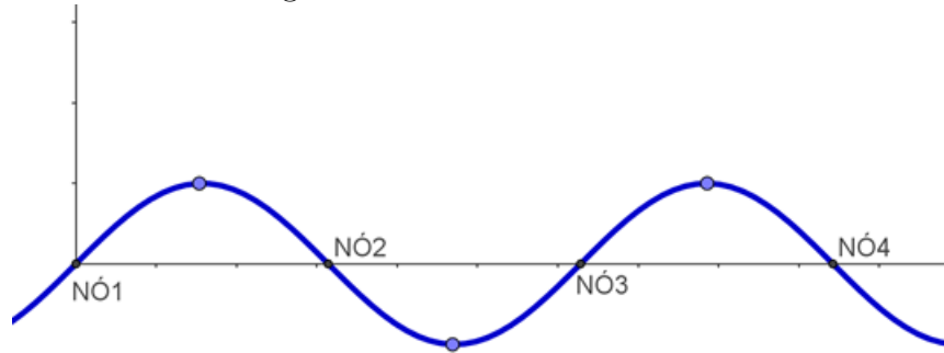
Figura 2.24: Onda harmônica.
