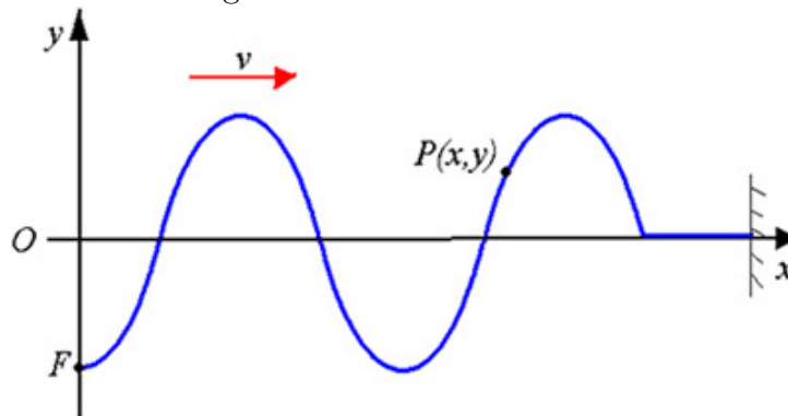
Figura 2.22: Onda senoidal.
