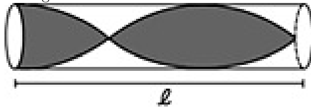
Figura 3.10: Tubo terceiro harmônico.
