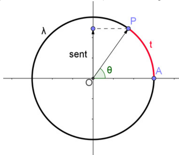
Figura 2.3: Circunferência \lambda , centrada no ponto O .
