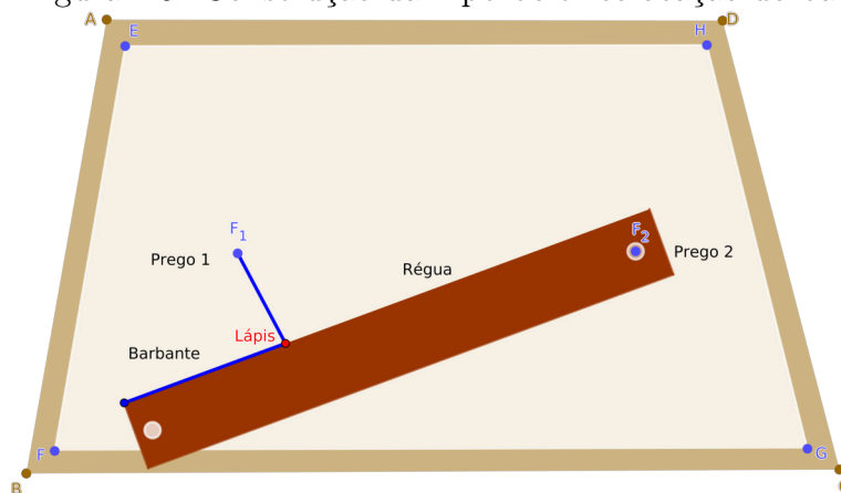
Figura 4.9: Construção da hipérbole: colocação do barbante
