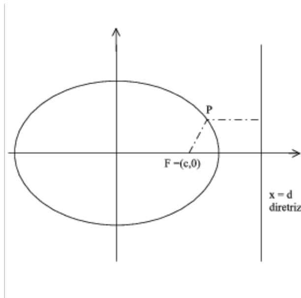
Figura 3.11: Cônica definida conforme a excentricidade
