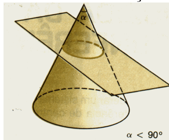
Figura 2.5: Elipse de Menaecmus: seção do cone acutângulo
