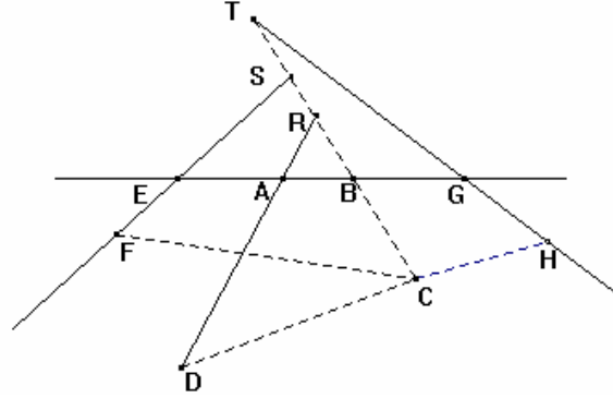
Figura 3.3: Problema de Pappus
