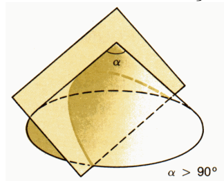
Figura 2.4: Hipérbole de Menaecmus: seção do cone obtusângulo
