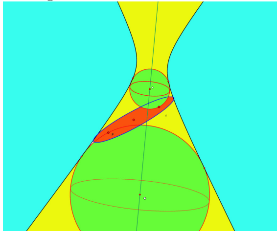
Figura 2.13: Esferas de Dandelin
