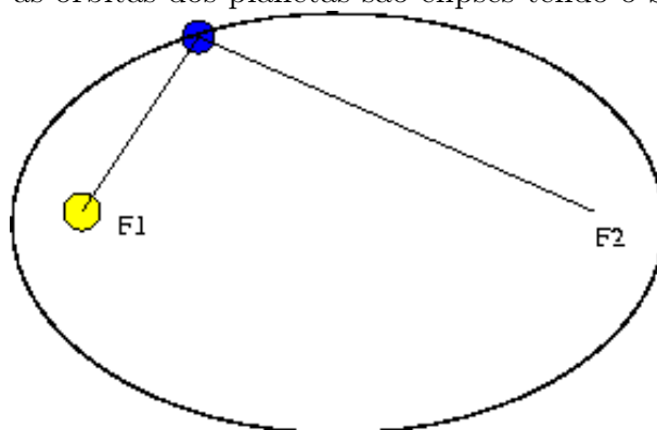
Figura 5.2: 1.a lei: as órbitas dos planetas são elipses tendo o Sol em um dos focos
