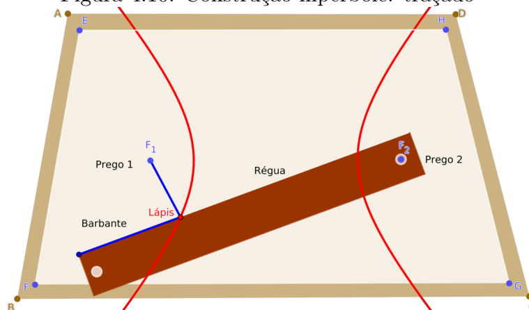
Figura 4.10: Construção hipérbole: traçado
