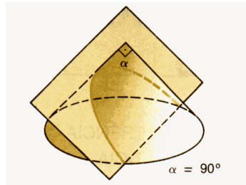
Figura 2.3: Parábola de Menaecmus: seção do cone reto
