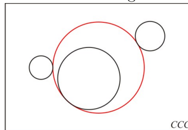
Figura 2.14: Problema original de Apolônio
