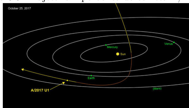
Figura 5.3: Trajetória hiperbólica do cometa A/2017 U1
