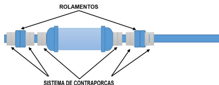
Figura 39: Eixo com os rolamentos colocados.
