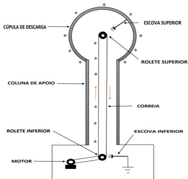
Figura 24. Esquema do GVDG
