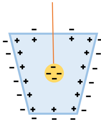
Figura 60: Separação das cargas elétricas do balde provocada pela presença da esfera eletrizada.
