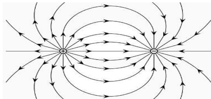
Figura 15: Configuração das linhas de força de um dipolo elétrico. Fonte: Disponível em: https://brasilecola.uol.com.br/fisica/linhas-forca.htm#
