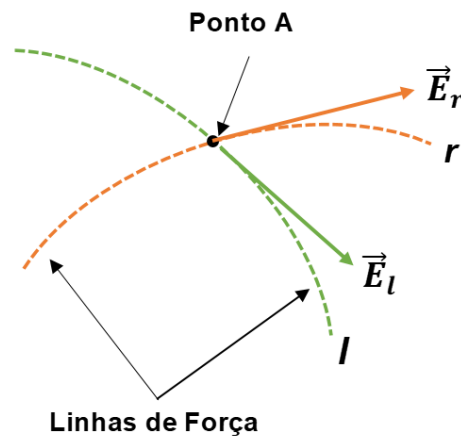
Figura 71: Cruzamento hipotético de duas linhas de força.
