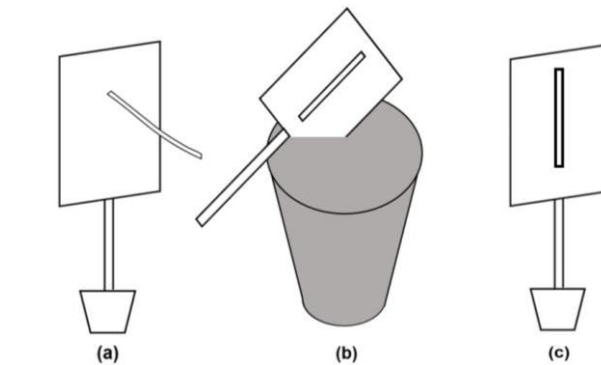
Figura 4: (a) Eletroscópio inicialmente carregado, ao entrar em contato com a água, descarrega-se (b). Ao ser retirado da água o eletroscópio se mantém descarregado (c).
