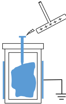
Figura 21: Capacitor sendo carregado pelo coletor de cargas do eletróforo. Mesmo sem o contato, as cargas são transferidas através do ar ionizado.:
