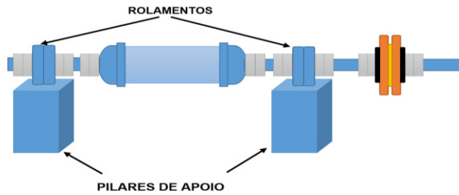
Figura 42: Eixo inferior apoiado sobre os pilares.
