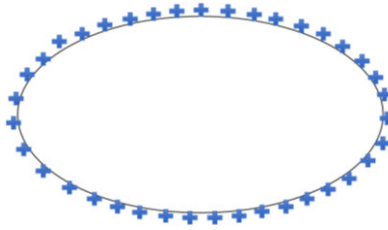
Figura 58: Cargas elétricas distribuídas na superfície de um condutor em equilíbrio eletrostático.
