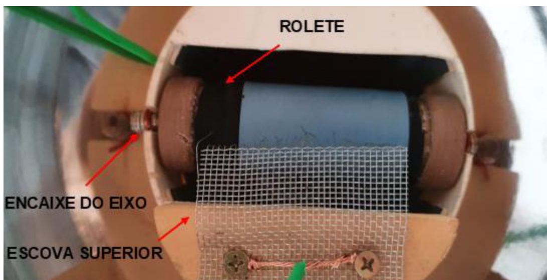
Figura 33: Roleta superior encaixado no cap superior.
