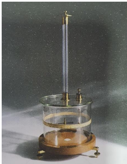
Figura 5 – Balança de torção apresentada por Coulomb em 1785 à Academia Francesa de Ciências
