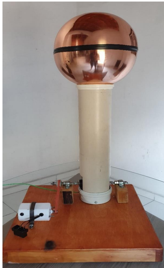
Figura 46: GVDG construído pelo autor.
