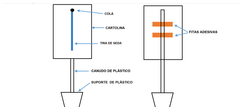
Figura 1: À esquerda a parte da frente do eletroscópio, e à direita a parte de trás.
