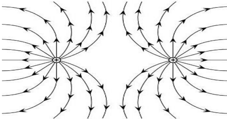
Figura 70: Configuração das linhas de força para dois eletrodos com cargas de mesmo sinal. Fonte: Disponível em: https://brasilescola.uol.com.br/fisica/linhas-forca.htm# .
