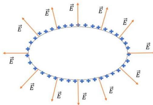
Figura 59: O campo elétrico é perpendicular à superfície do condutor em equilíbrio eletrostático.
